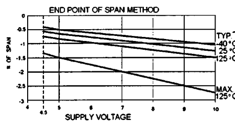
线性度 VS V_s
