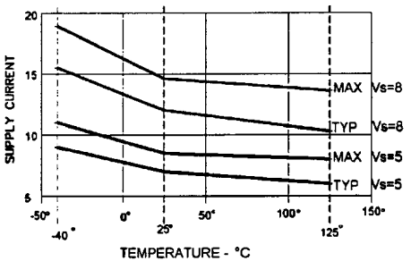
供电电流 VS 温度
